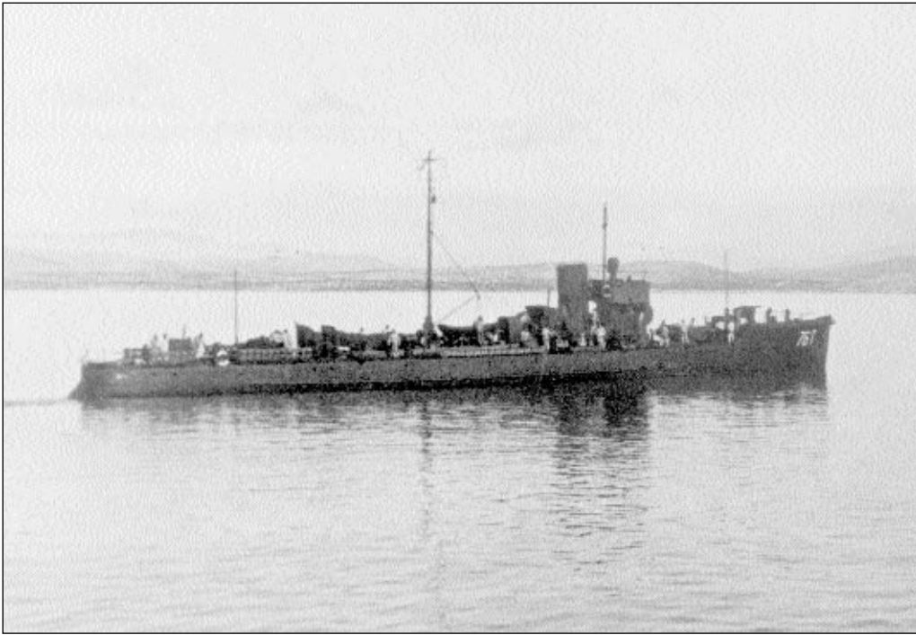
(293) Torpedoboot 76
